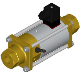
Stellungsanzeige position indication elektrische Option = 19 electrical option = 19
