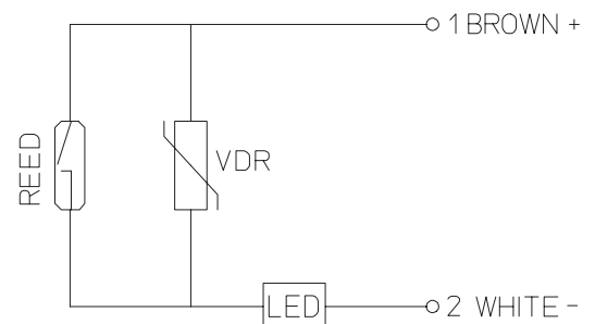
Schema elettrico dei finecorsa Limit-switch electric plan
